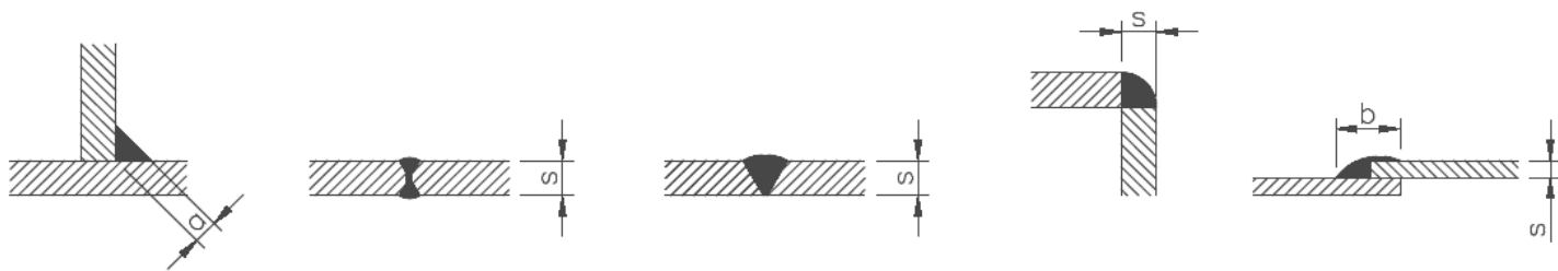
Kehl-naht A - Schuh Doppel V-Naht DV - Schuh V-Naht V - Schuh Ecknaht E - Schuh Überlappnaht U - Schuh
